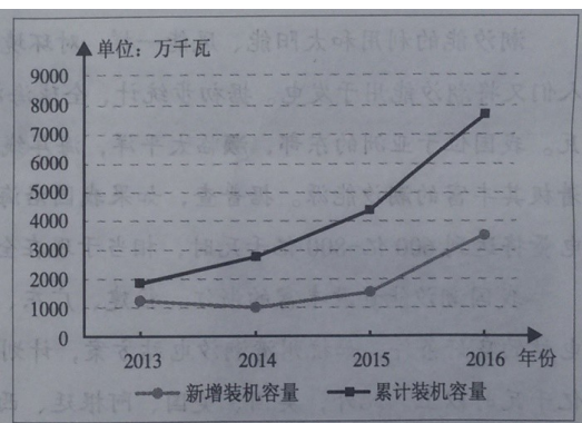
中国光伏发电装机容量统计图
